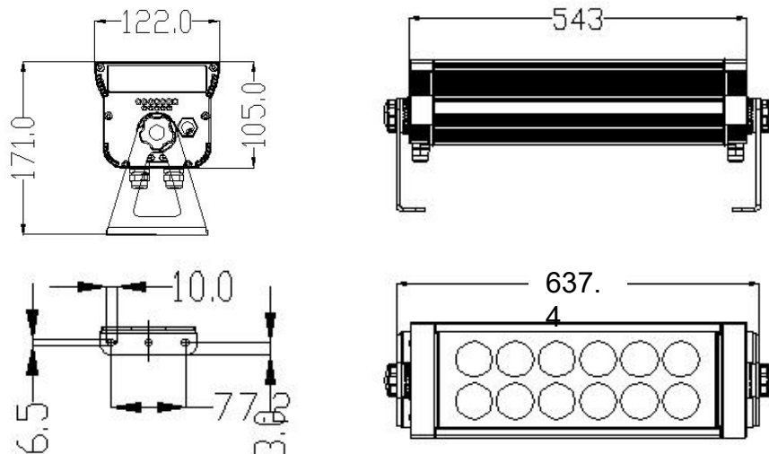
安装底板尺寸图
